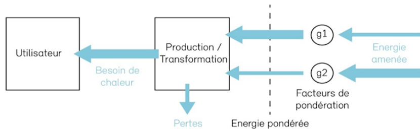
Illustration 28 : Réseaux anergie
