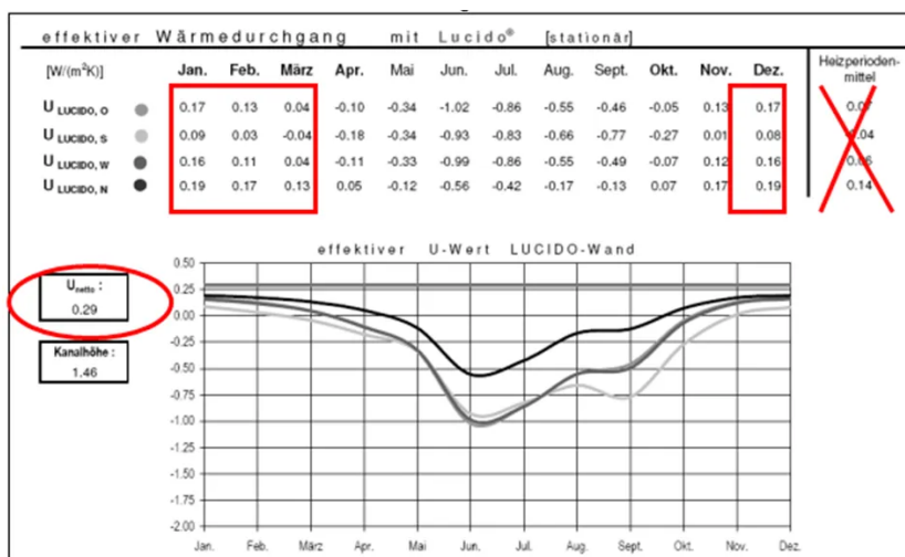
Illustration 9 : détermination de la valeur U pour le système de façade Lucido
