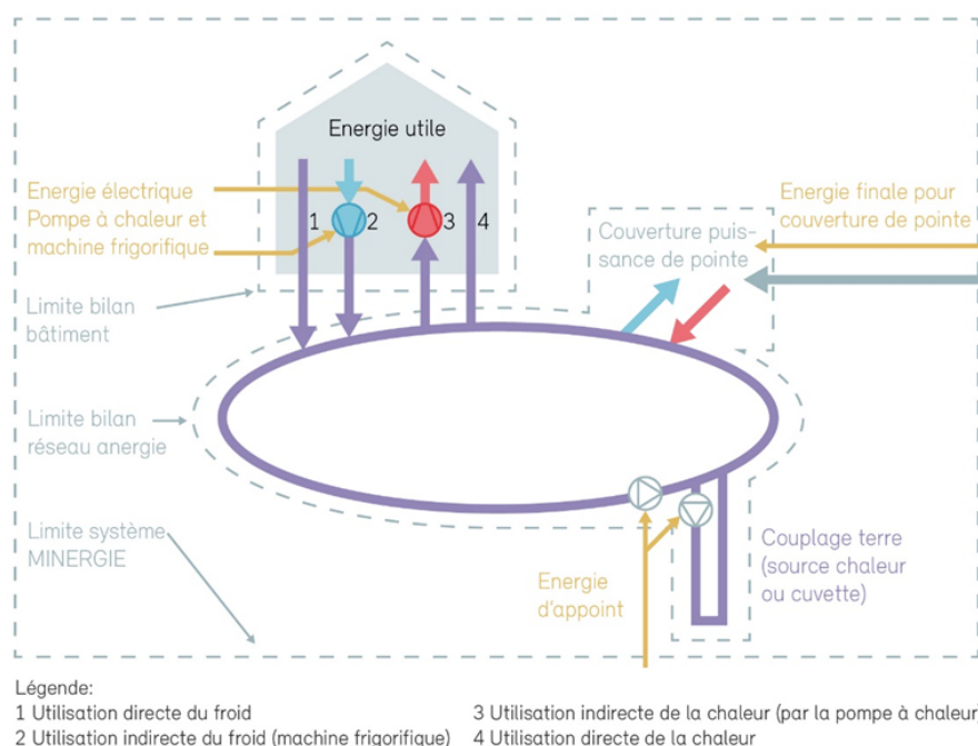
Illustration 27 : Réseaux énergie
