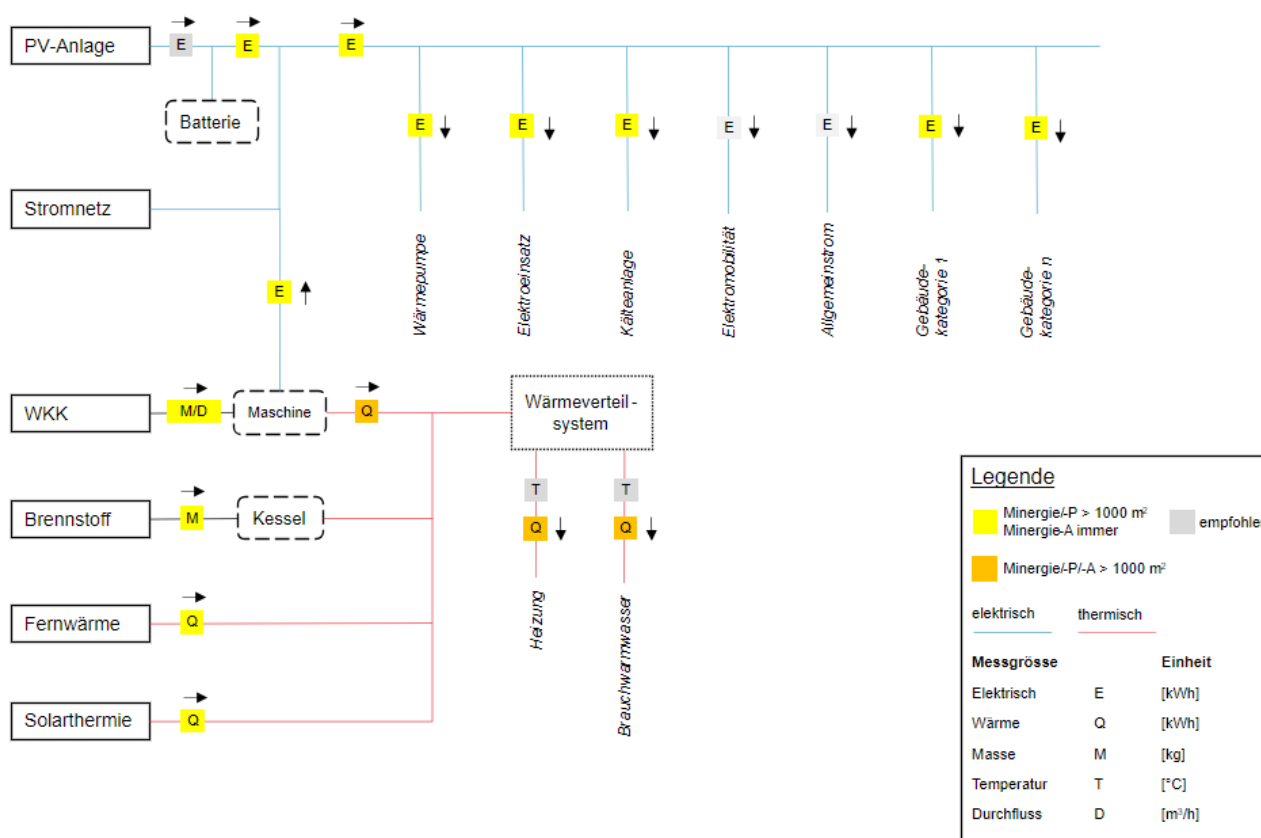
Illustration 43 : Exemple de points de mesure pour un immeuble avec chauffage par pompe à chaleur et corps de chauffe électrique pour la production d'eau chaude sanitaire
