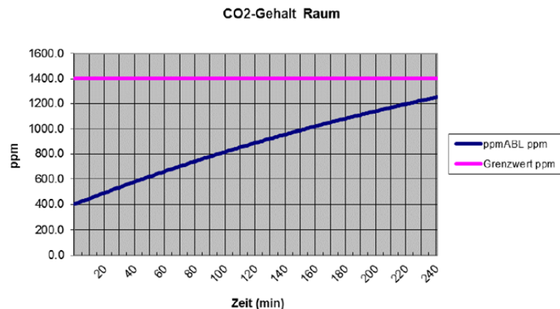
Illustration 33 : Teneur en CO 2 pour deux personnes
