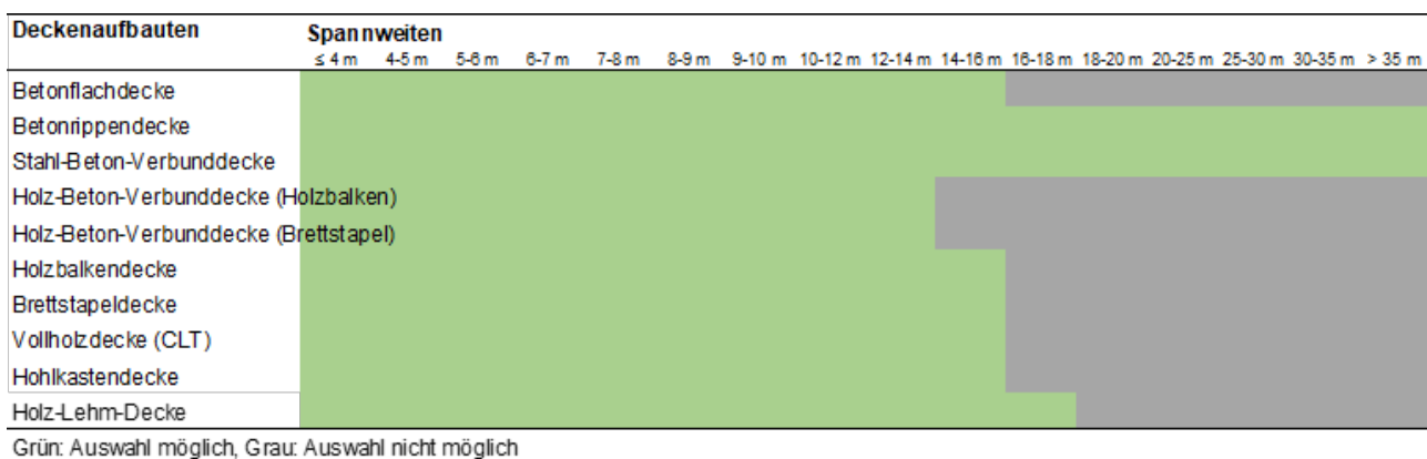
Abbildung 48: zeigt die möglichen Kombinationen zwischen Spannweite der Tragstruktur der Decke und Deckenaufbauten. Grün = Auswahl möglich, Grau = Auswahl nicht möglich.
