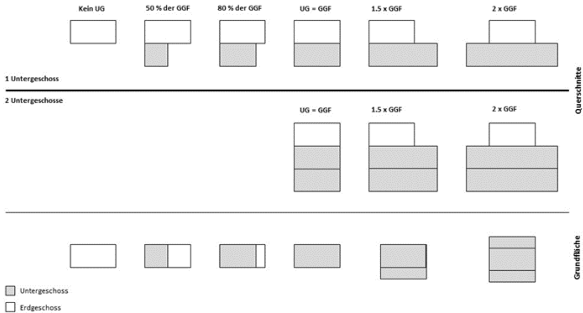
Abbildung 46: bildet die neun verschiedenen Eingabemöglichkeiten der Eingabe "UG-Gestaltung" ab
