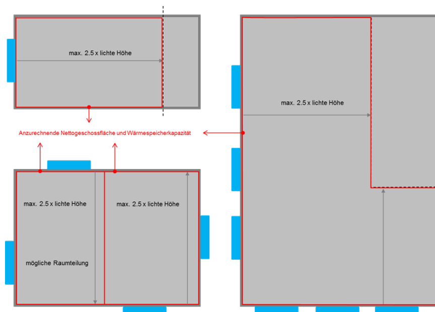
Abbildung 17: maximale anzurechnende Raumtiefe und Aufteilung von Räumen
