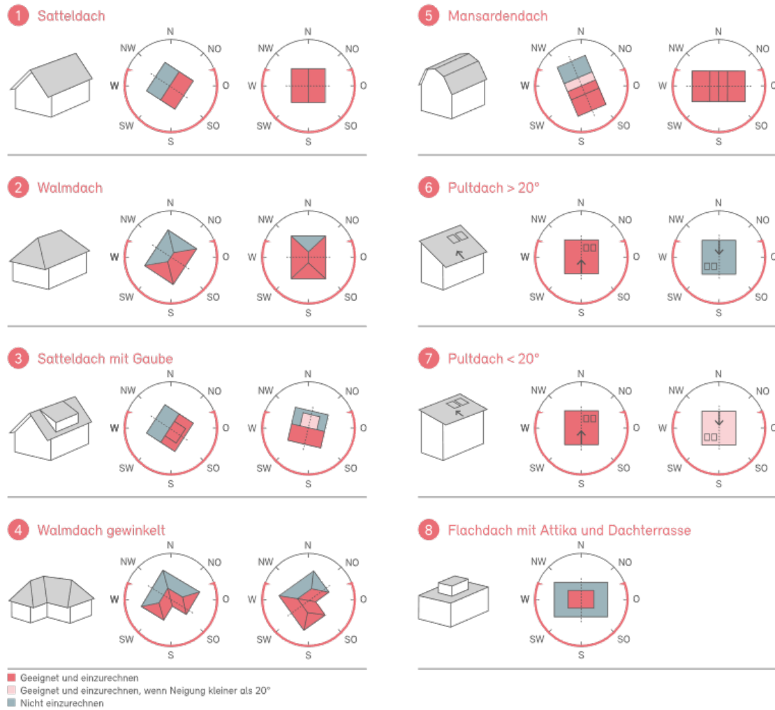
Abbildung 40: Einrechnung der nutzbaren Dachfläche anhand einiger Beispieldächer.
