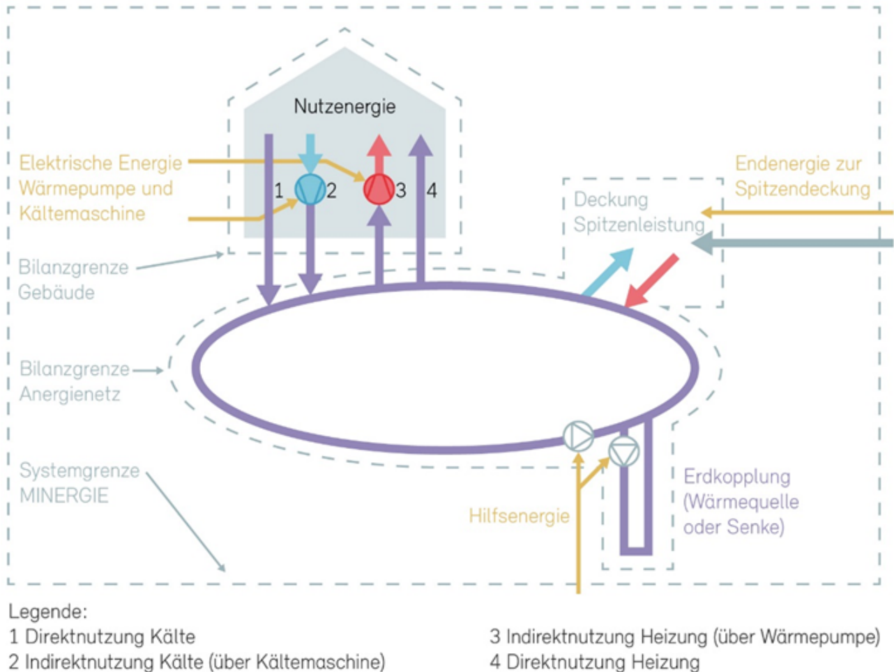
Abbildung 25: Prinzipskizze Anergienetz
