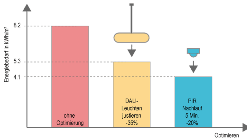
Abbildung 35: Beispiel «Optimierung Beleuchtung in einem Schulhaus»
