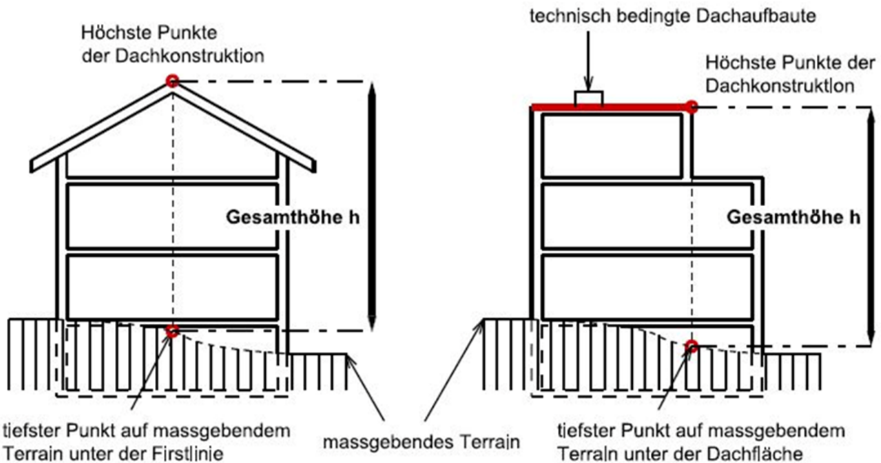
Abbildung 3: Definition Gesamthöhe Gebäude
