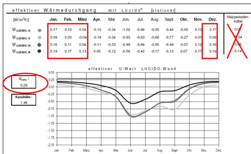
Abbildung 9: Festlegung U-Wert bei Lucido Fassadensystem
