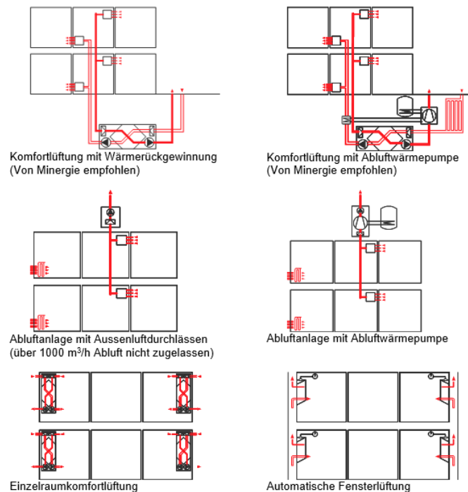
Abbildung 29: Auswahl Lüftungsanlagen für «Standard-Lüftungsanlagentyp»
