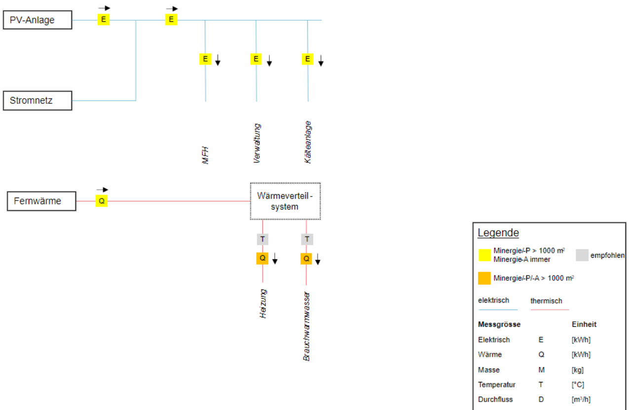
Abbildung 45: Datenpunkte Minergie Monitoring am Beispiel MFH und Verwaltung mit Fernwärme und Kühlung
