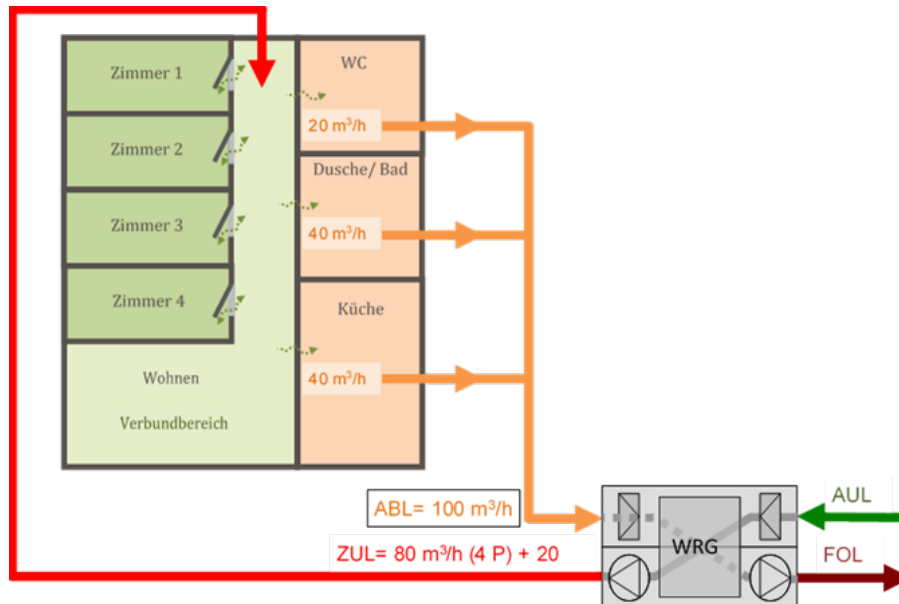
Abbildung 32: Beispiel Grundlüftung für Erneuerungen
