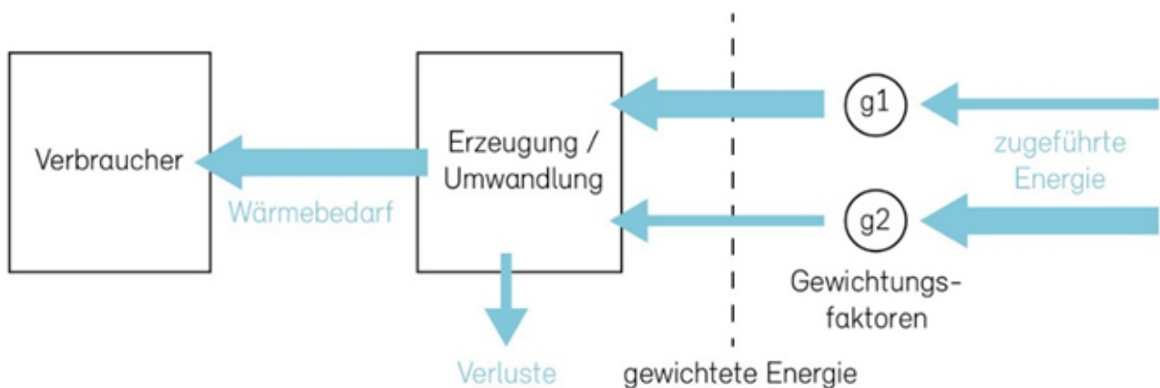
Abbildung 26: Prinzip der Energieberechnung im Minergie-Standard
